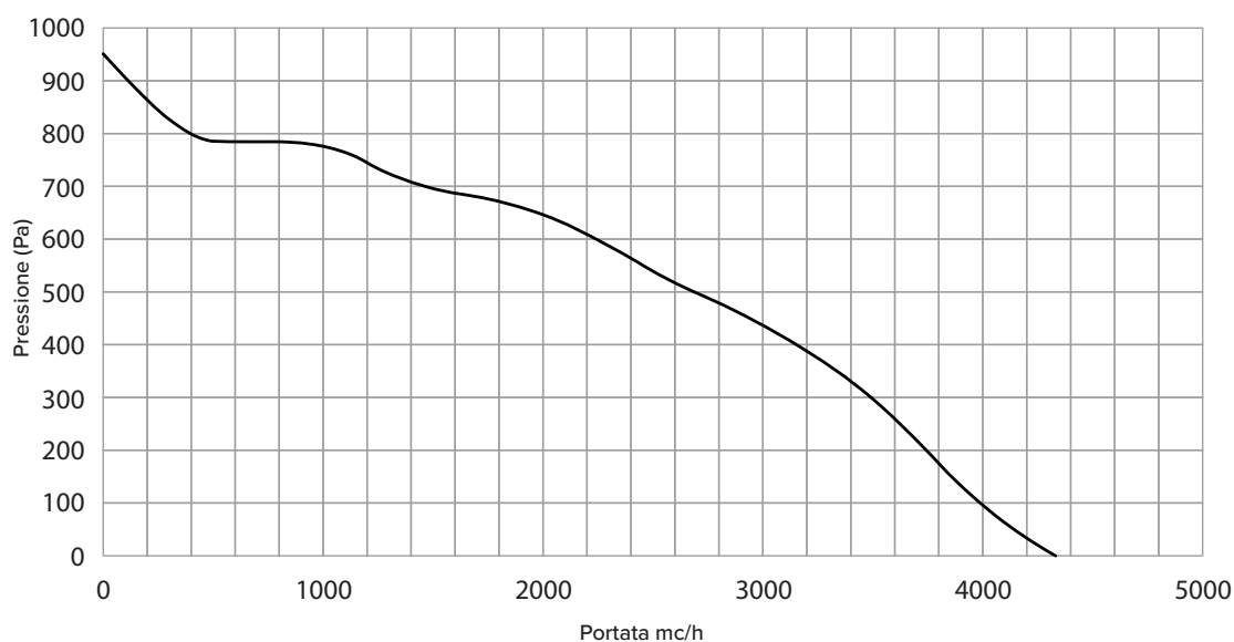
VORT ANTIFUMO 4000 EVO Cod.90029
