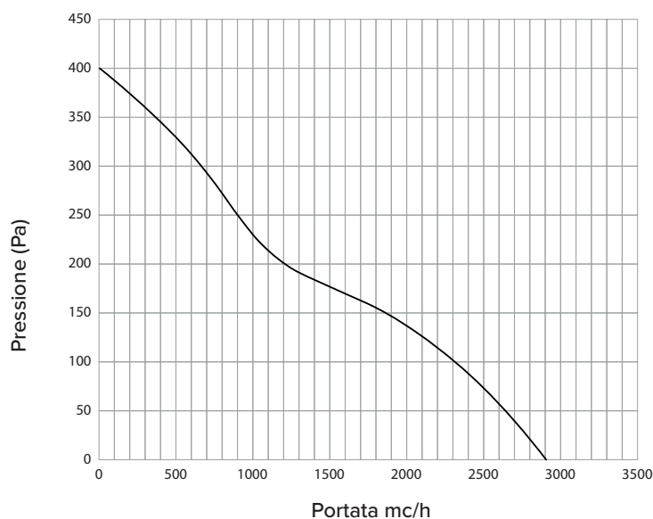
PREVALENZA VENTILATORE VORT ANTIFUMO 3000 Cod.90025
