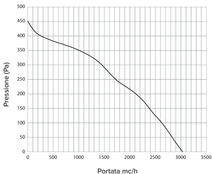
PREVALENZA VENTILATORE VORT ANTIFUMO 3000 EVO Cod.90028
